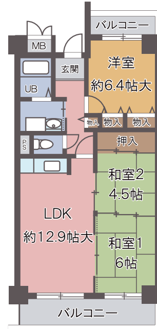
F 3LDK type 67.62㎡ ■バルコニー面積/12.81㎡ ※CタイプはFタイプの反転となり、バルコニーの形状が異なります。
