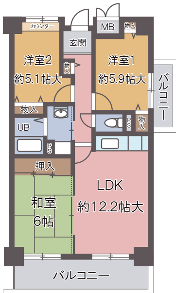
B 3LDK type 67.50㎡ ■バルコニー面積/13.18㎡ ※AタイプはBタイプの反転となります。
