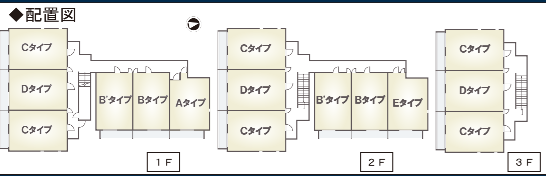
C type 1LDK ■専有面積 / 36.43㎡ ■101.201.301は反転となります。
